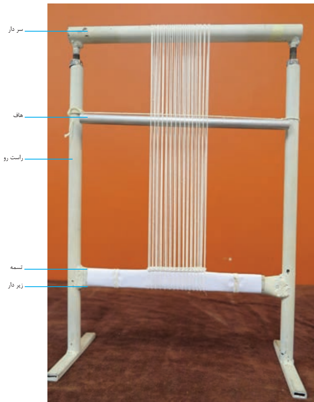
▲ تصویر ۱-۳۰ چله کشی شده و اجزای آن
