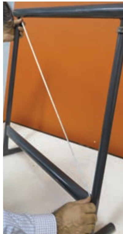
تصویر ۱-۱۱ اندازه گیری فاصله نقاط میانی راست روها
